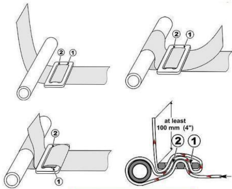
Крепление ремней с "плоской пряжкой"
