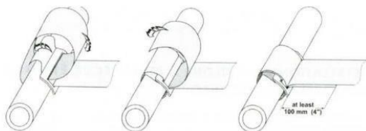
Крепление ремней с "вогнутой пряжкой"
